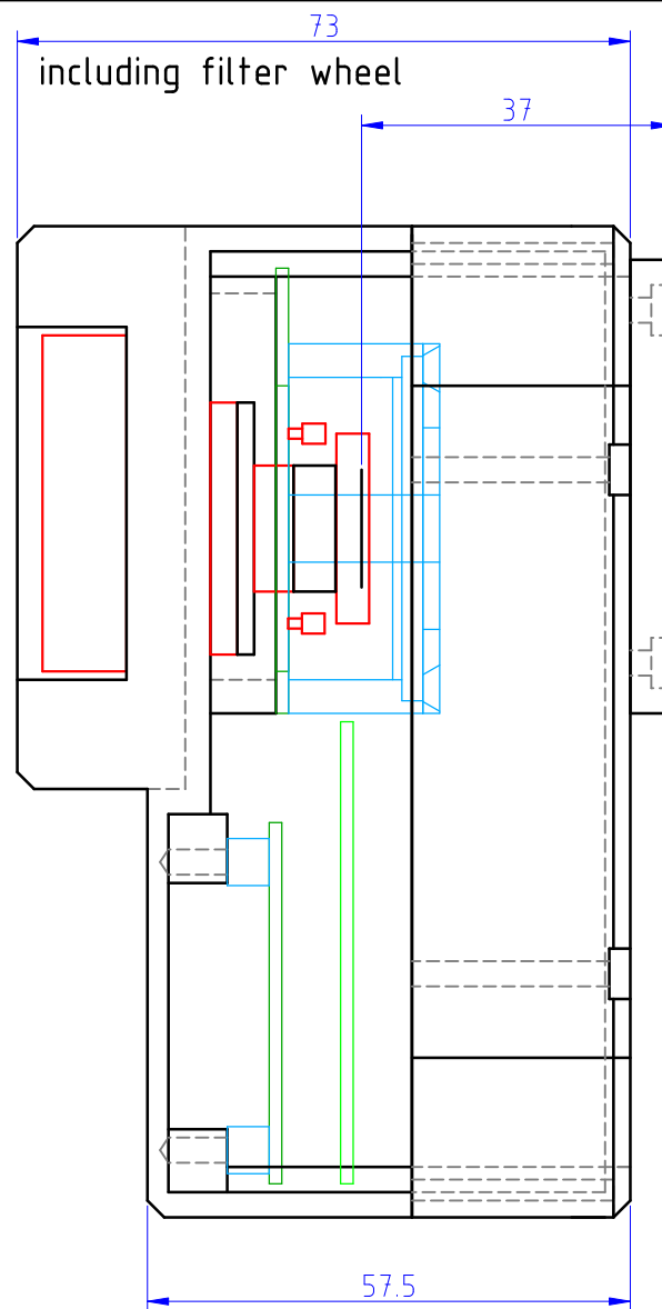
ASTROELEKTRONIK FISCHER SIGMA2 - Auflagemaß - back focus
